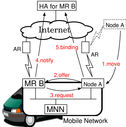
図 5: 計算機を移動ルータとして動的に追加する機構
