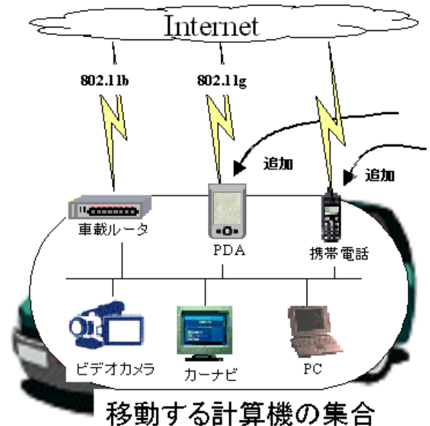
図2: 移動する計算機群のインターネット接続性を動的に共有する例
