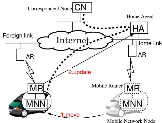
図 3: Network Mobility の移動透過処理
