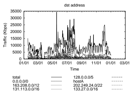
図 4.4: データ A destination ip address
