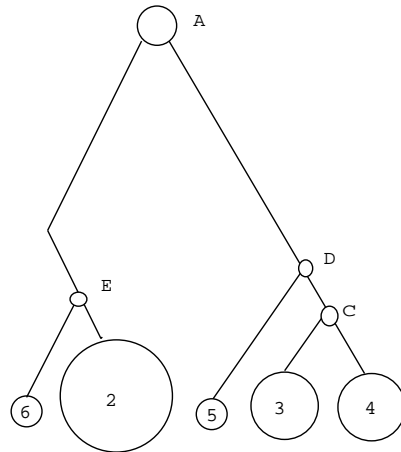
図 3.8: パトリシアツリーへの LRU を用いたデータの追加 2
